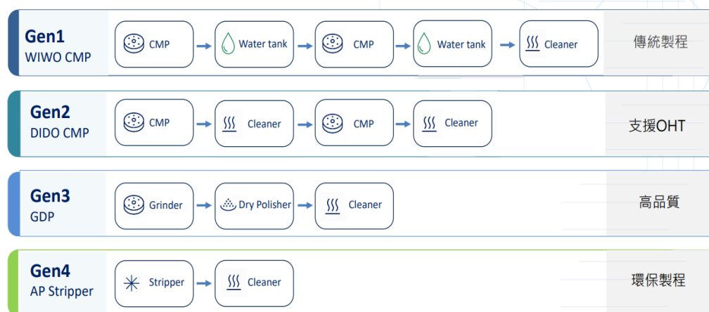
圖表五：再生晶圓 Gen1~4 技術演進示意圖
