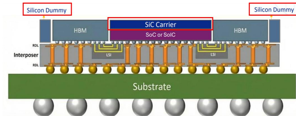
圖表七：公司先進封裝解決方案應用點(如下圖紅框處)
